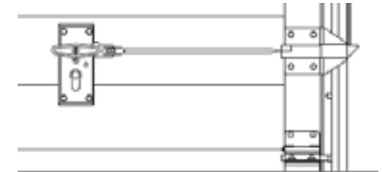
Standaard enkelzijdige vergrendeling met europrofiel cilinder
