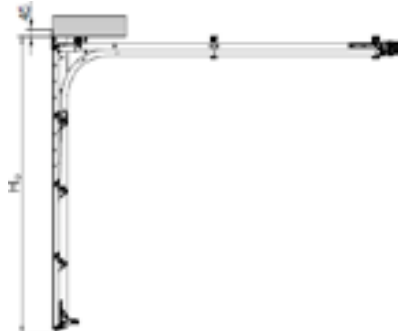
Verticale doorsnede, montage IN de opening, afwerking voor de opening
