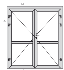
MB60 systeem aluminium dubbele deur met thermische onderbreking
