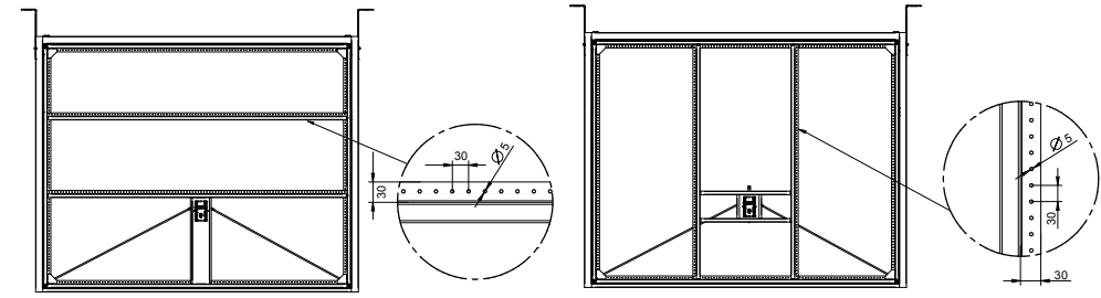
Garagedeur Komfort voor een individuele vulling - verticaal
