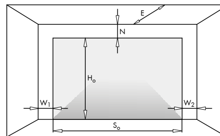
Maatvoering en zijruimtes benodigd voor installatie
