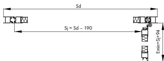
Installatie in de opening - horizontaal - enkele deur AW45 systeem
