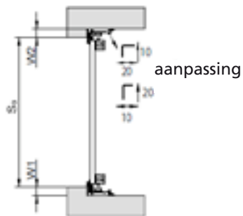
Horizontale doorsnede, montage achter de opening
