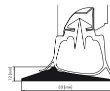
Afdichtingsdrempel
