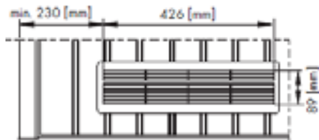
K1 Rooster Standaard kleuren: RAL 9005 – 9016 – 8014 – 8017
