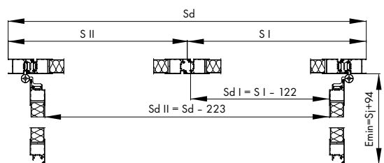
Installatie in de opening - horizontaal - Dubbele deur AW45 systeem
