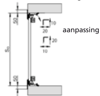
Horizontale doorsnede, montage IN de opening, afwerking voor de opening
