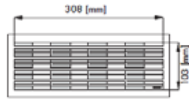
K3 Rooster Standaard kleuren: RAL 9005 – 9016 Voorzien van verstelbare lucht doorvoer en gaas
